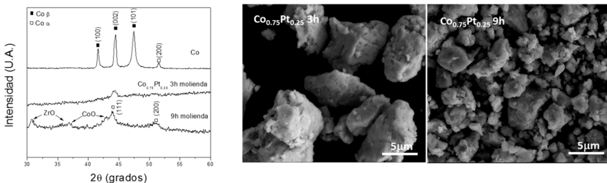
Figura 2. Resultados de caracterización del electrocatalizador de \text{Co}_{0.75}\text{Pt}_{0.25} : Izq. Resultados de difracción de rayos X en diferentes tiempos de molienda. Der. Imágenes de microscopía electrónica de barrido en diferentes tiempos de molienda.
