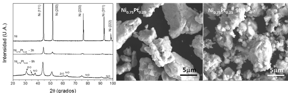
Figura 1. Resultados de caracterización del electrocatalizador de Ni_{0.75}Pt_{0.25} : Izq. Resultados de difracción de rayos X en diferentes tiempos de molienda. Der. Imágenes de microscopía electrónica de barrido en diferentes tiempos de molienda.
