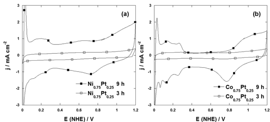
Figura 4. Voltamogramas de los electrocatalizadores obtenidos: a) \text{Ni}_{0.75}\text{Pt}_{0.25}/\text{C} y b) \text{Co}_{0.75}\text{Pt}_{0.25}/\text{C} . Datos obtenidos en 0.5\text{M H}_2\text{SO}_4 a 25^\circ\text{C} con una velocidad de barrido de 50\text{ mV s}^{-1} .
