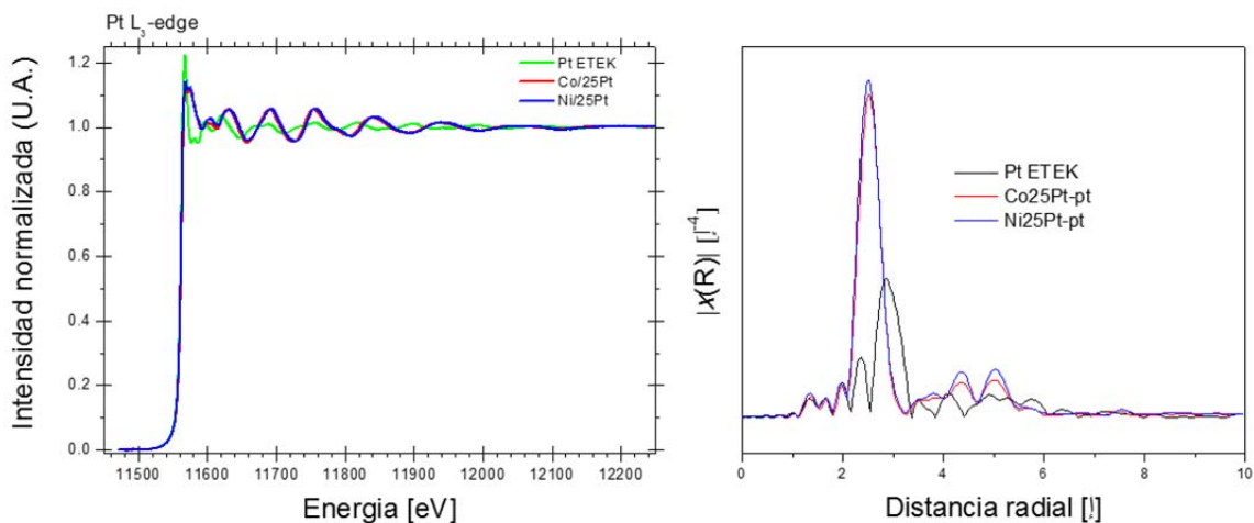
Figura 3. Resultados de caracterización por espectroscopia de absorción de rayos X de los electrocatalizadores obtenidos después de 9 horas de molienda.
