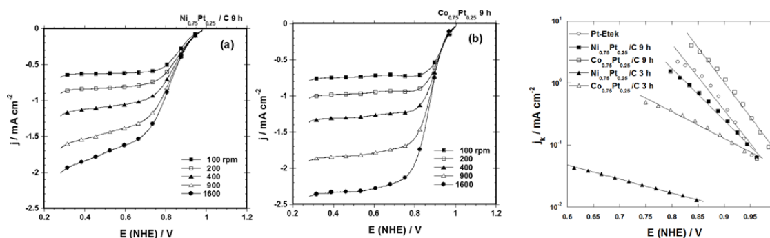
Figura 4. Voltamogramas de los electrocatalizadores obtenidos: a) \text{Ni}_{0.75}\text{Pt}_{0.25}/\text{C} ; b) \text{Co}_{0.75}\text{Pt}_{0.25}/\text{C} . Datos obtenidos en 0.5\text{M H}_2\text{SO}_4 a 25^\circ\text{C} con una velocidad de barrido de 50\text{ mV s}^{-1} . c) Gráficos de Tafel corregidos por transferencia de masa deducidos del análisis de EDR del oxígeno saturado 0.5\text{ M H}_2\text{SO}_4 a 25^\circ\text{C} .
