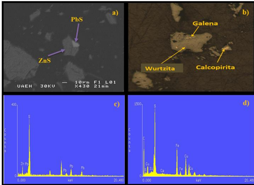
Figura 5. a) Micrografía obtenida con electrones retrodispersados a 430X. b) Micrografía óptica obtenida con nicóles cruzados a 10X. c) Espectro de energías dispersivas de Rayos X mostrando la presencia de S, Zn y Pb. d) Espectro de energías dispersivas de Rayos X mostrando la presencia de S, Cu, Fe, Si y Ca.
