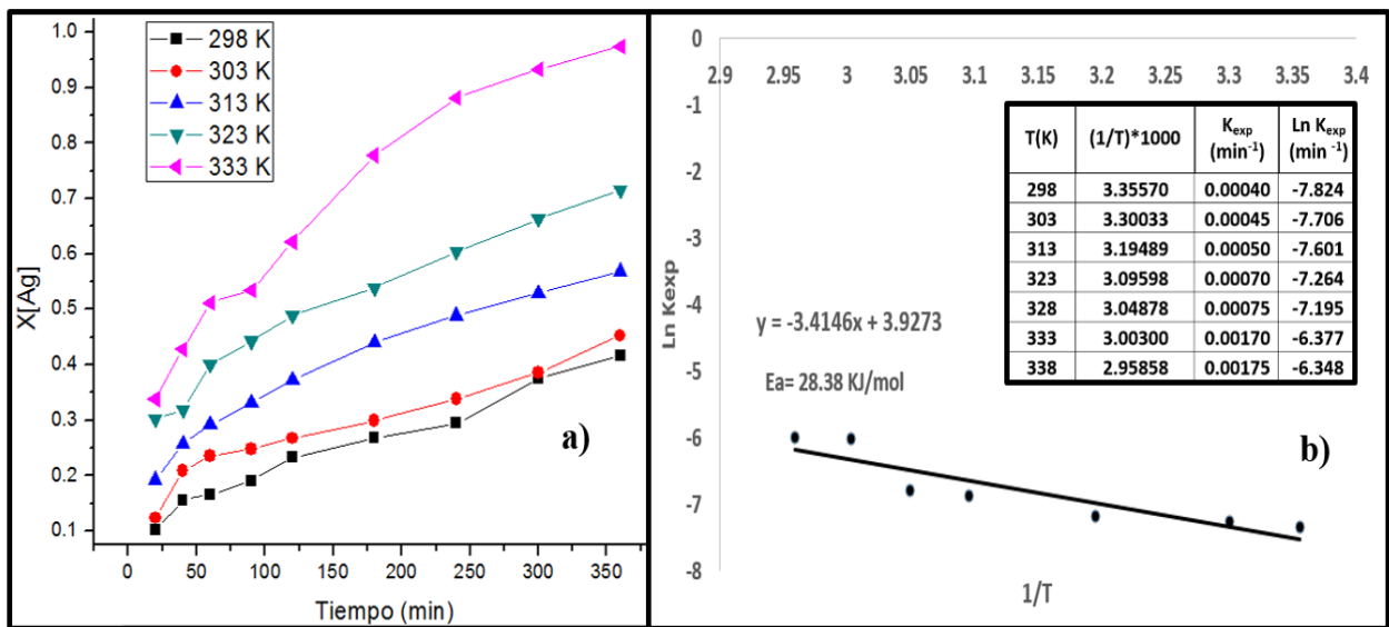
Figura 7. a) Representación gráfica del efecto temperatura a 298, 303, 313,323 y 333 K. b) Dependencia de K exp en función de la temperatura. Energía de Activación=28.38 KJ.
