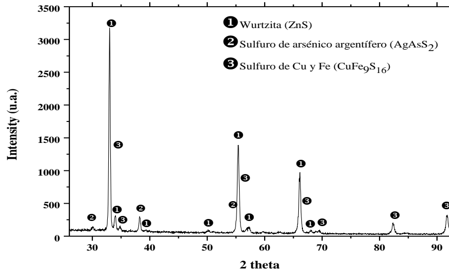
Figura 3. Difractograma de rayos X de los polvos del concentrado de Zn.
