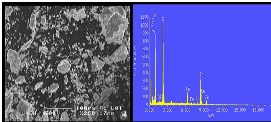
Figura 4. Micrografía del concentrado de Zn obtenida a 250 X muestra la morfología de las partículas y el análisis EDS.
