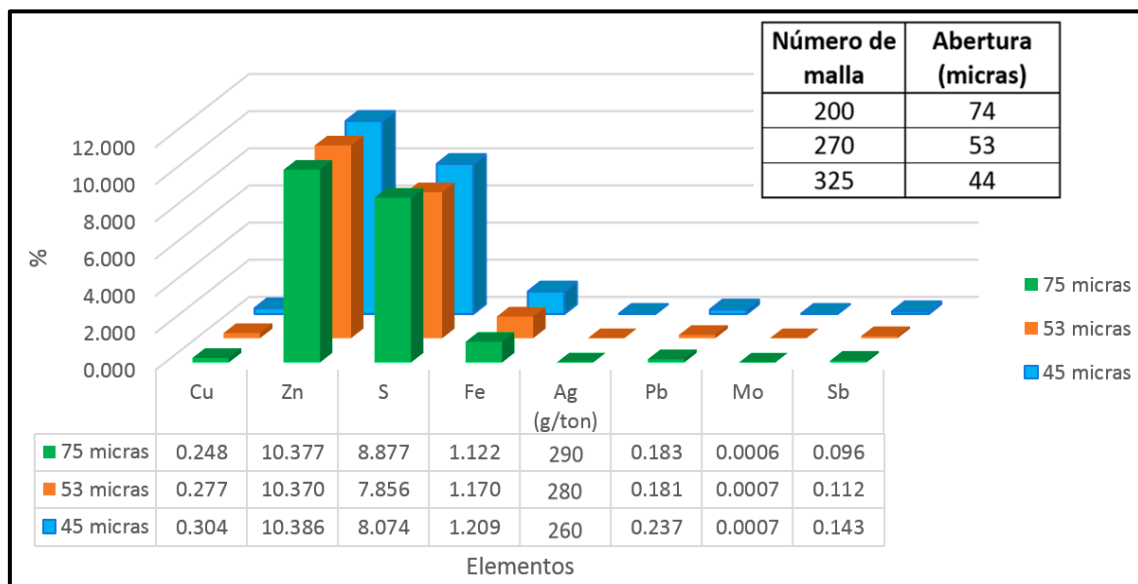
Figura 1. Composición química en porcentaje del concentrado de Zn a diferentes tamaños de partícula.
