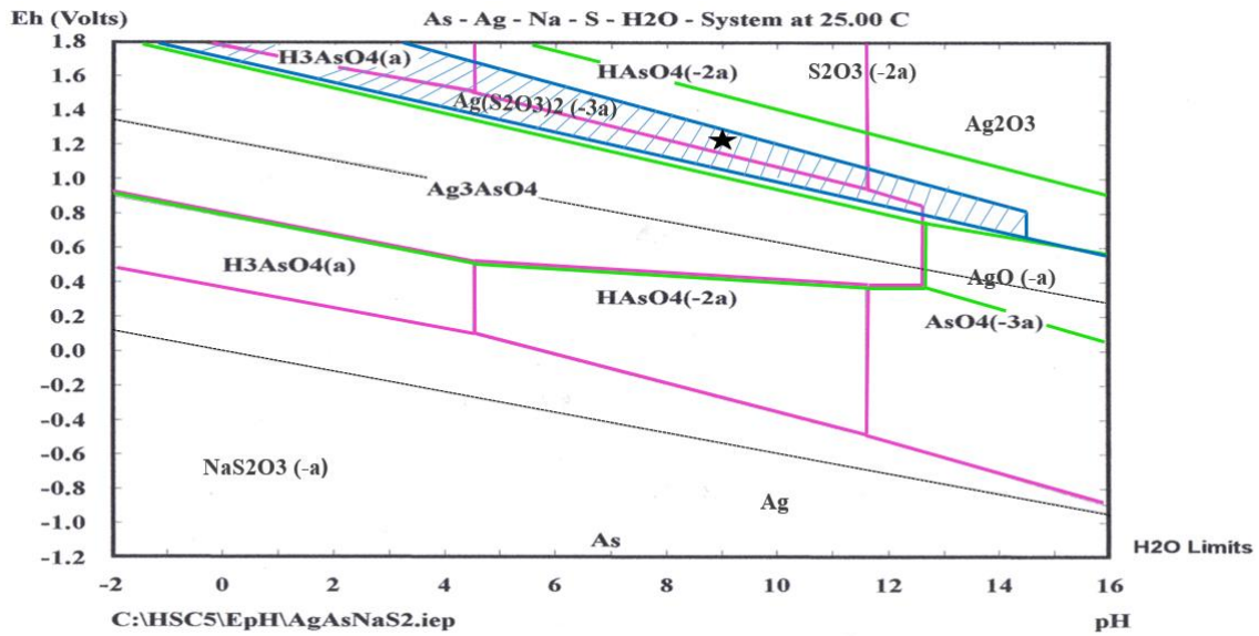
Figura 6. Diagrama eh-pH para el sistema Ag-As-Na-H 2 O a 298.15 K
