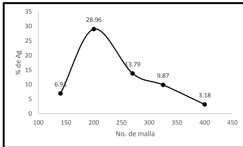
Figura 2. Distribución de Ag (%) con respecto al número de malla.
