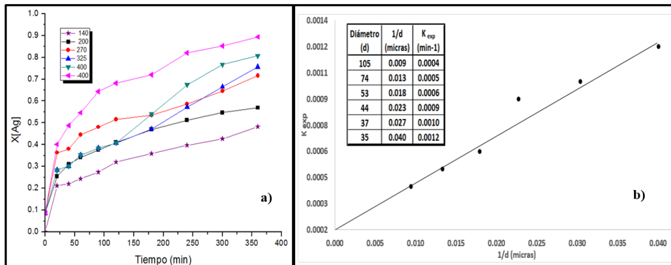
Figura 8. a) Representación gráfica del efecto tamaño de partícula. b) Dependencia de K exp en función del inverso del diámetro de partículas.
