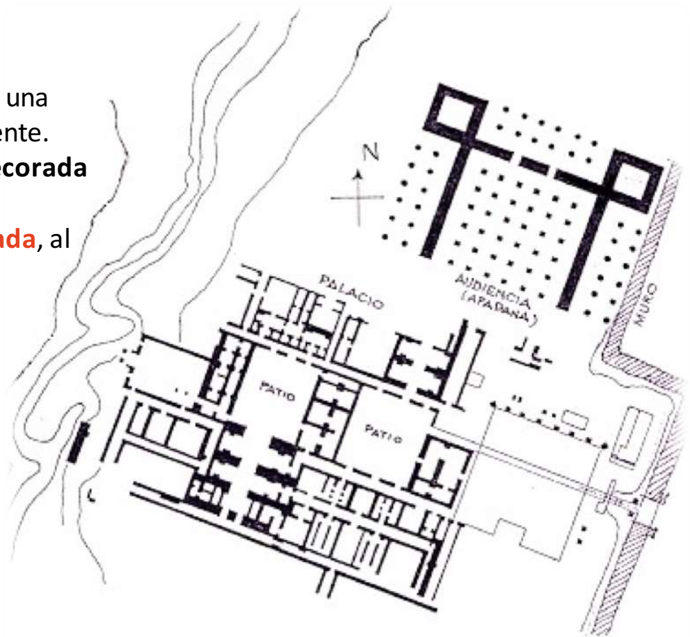
Planta del Palacio y de la Apadana de Susa.
