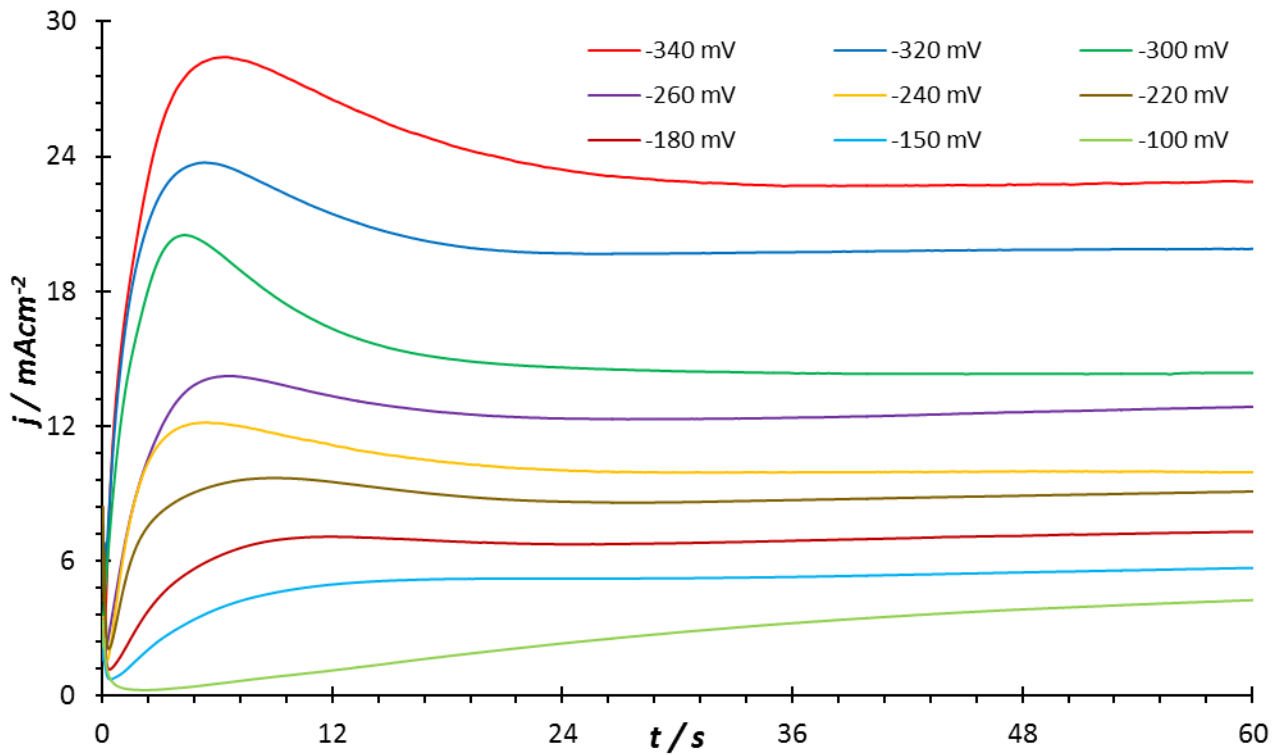
Figura 4.15 Transitorios obtenidos mediante el trazado de pico de corriente vs tiempo en un rango de potencial de 0 a -400 mV a partir del sistema I a 35°C.
