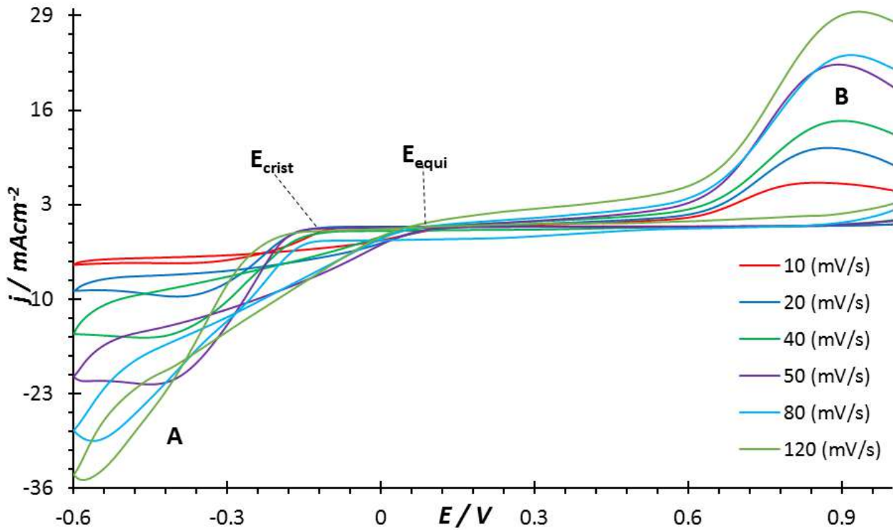
Figura 4.4 Voltamperograma cíclico típico obtenido a partir del sistema I, a diferentes velocidades de barrido a 35^\circ\text{C} .
