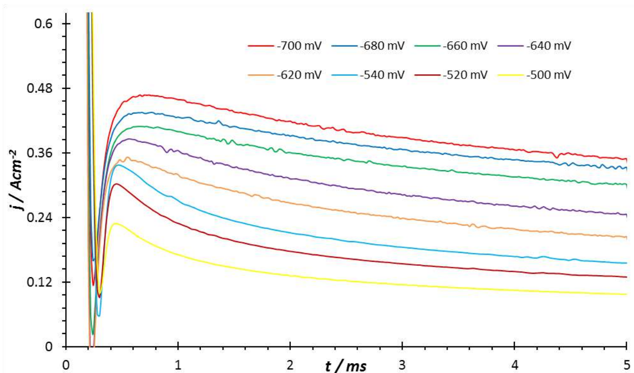
Figura 5.8 Transitorios obtenidos mediante el trazado de pico de corriente vs tiempo en un rango de potencial de -300 a -700 mV a partir del sistema I a 25°C utilizando un UME de 25 \mu\text{m} de diámetro.
