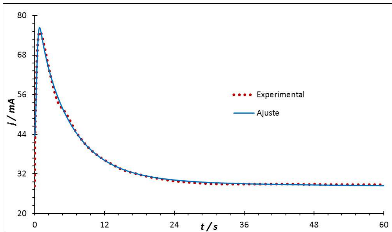
Figura 4.26 Ajuste de un cronoamperograma con potencial de -300 mV mediante el sistema I a 40°C, utilizando el modelo matemático de Palomar–Pardavé et al.
