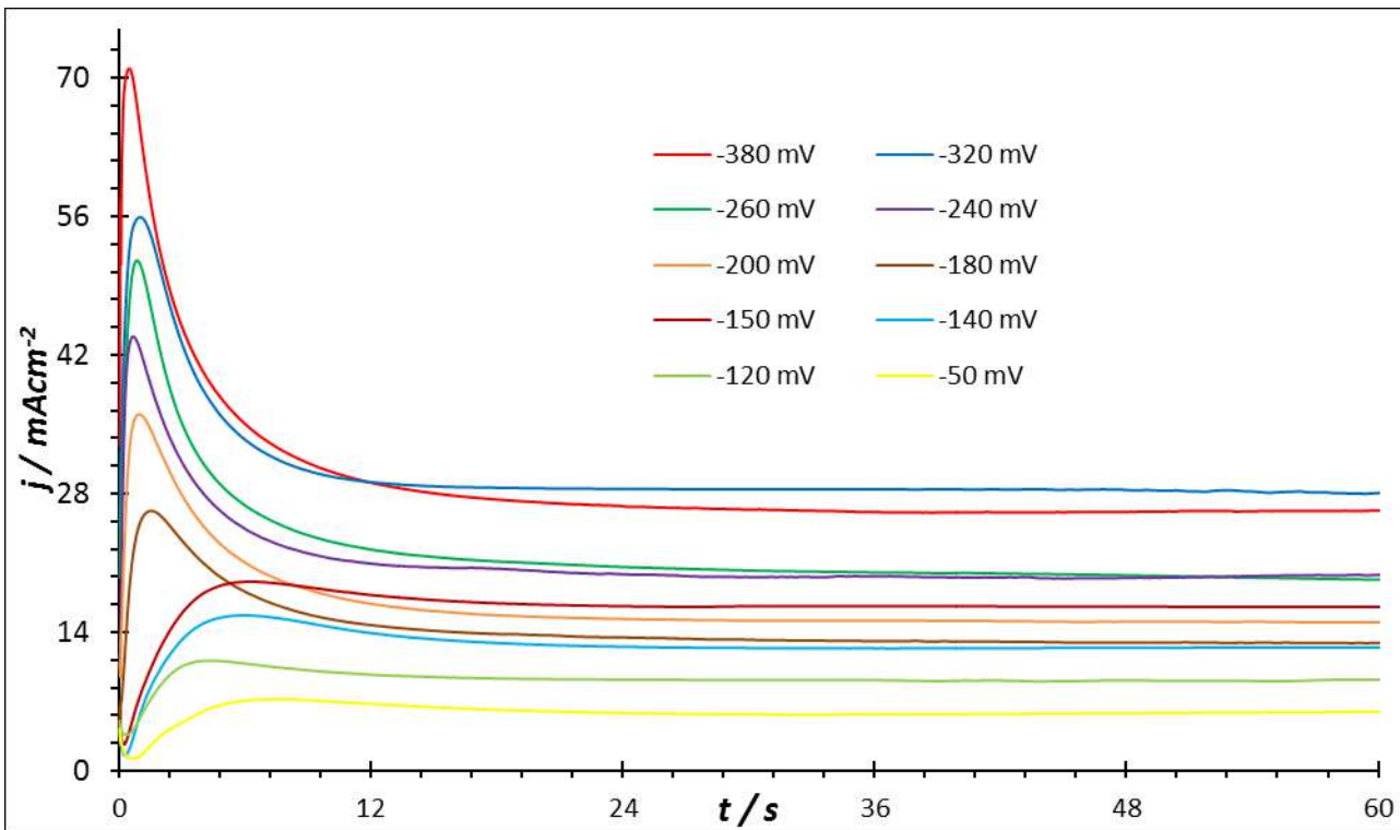
Figura 4.16 Transitorios obtenidos mediante el trazado de pico de corriente vs tiempo en un rango de potencial de 0 a -400 mV a partir del sistema I a 40°C.
