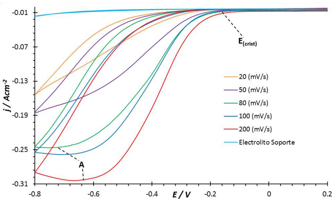
Figura 5.2 Voltamperograma cíclico típico obtenido a partir de los sistema I y II, utilizando un UME de 15 µm de diámetro, con diferentes velocidades de barrido a 25°C.
