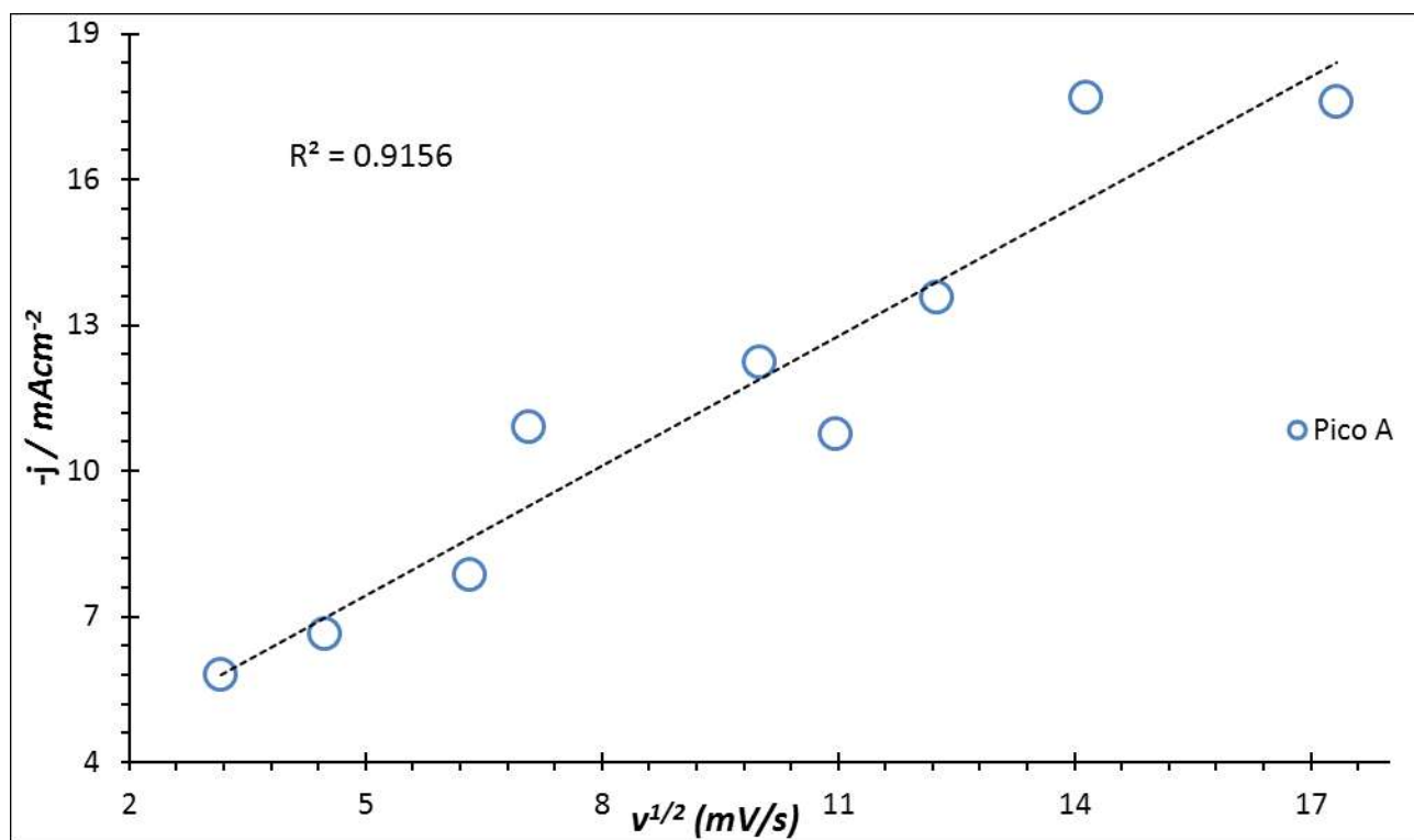
Figura 4.12 Gráfica de la corriente de pico vs v^{1/2} del sistema I a 25°C.
