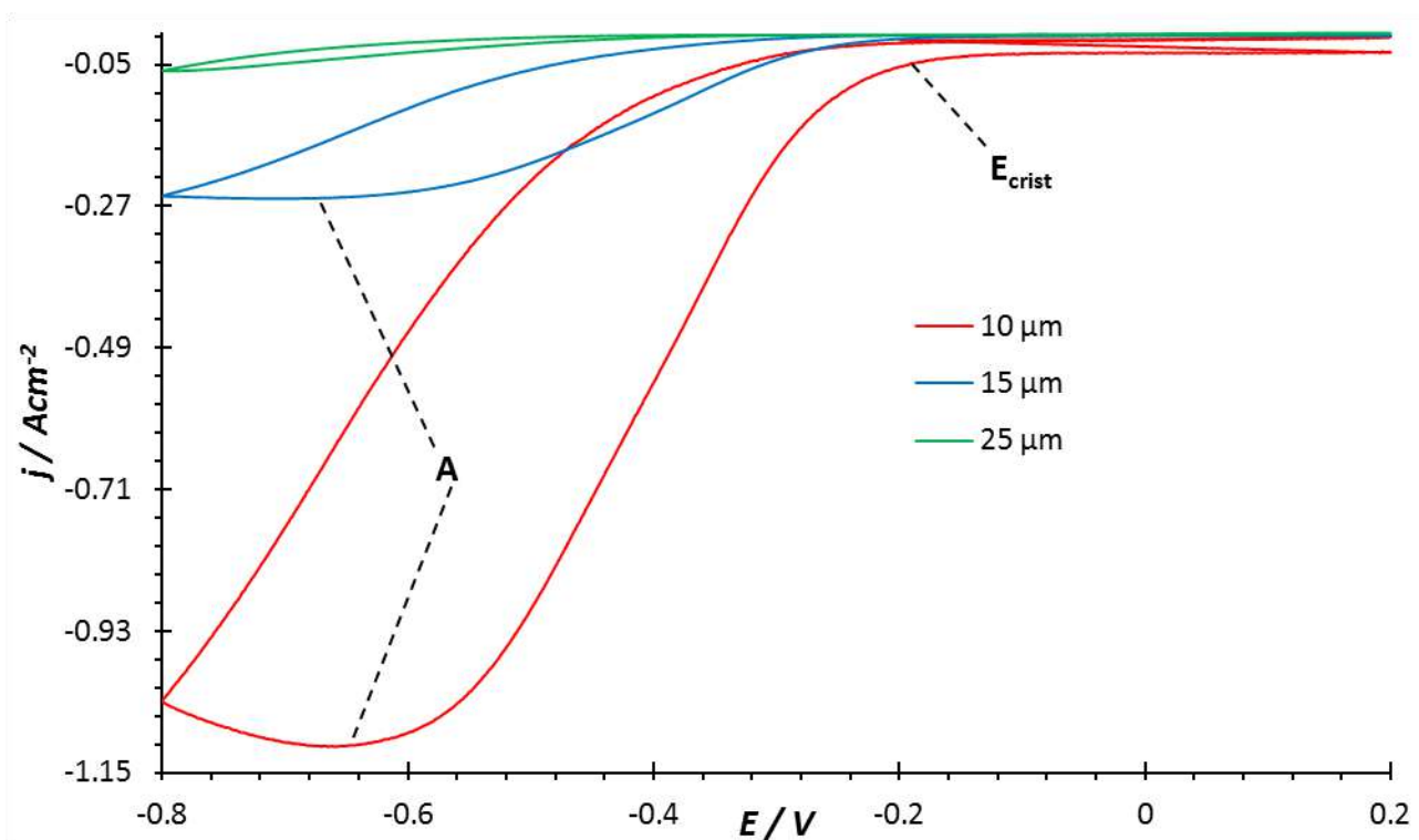
Figura 5.4 Voltamperograma cíclico típico obtenido a partir del sistema I, utilizando UMEs de diferentes diámetros, a una velocidad de barrido de 70 \text{ mV s}^{-1} y a una temperatura de 25^\circ\text{C} .
