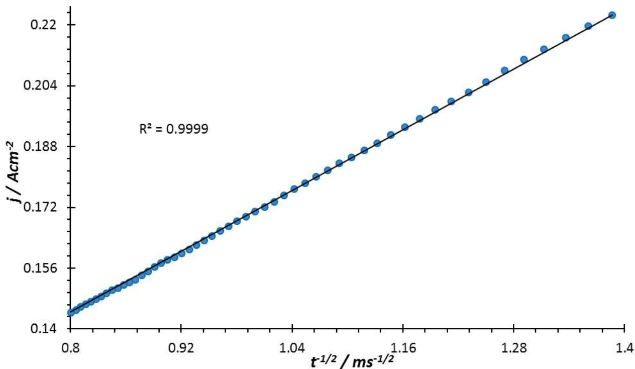
Figura 5.9 Gráfica de la corriente de pico vs t^{1/2} / \text{s}^{-1/2} de acuerdo a la ecuación de Cottrell.
