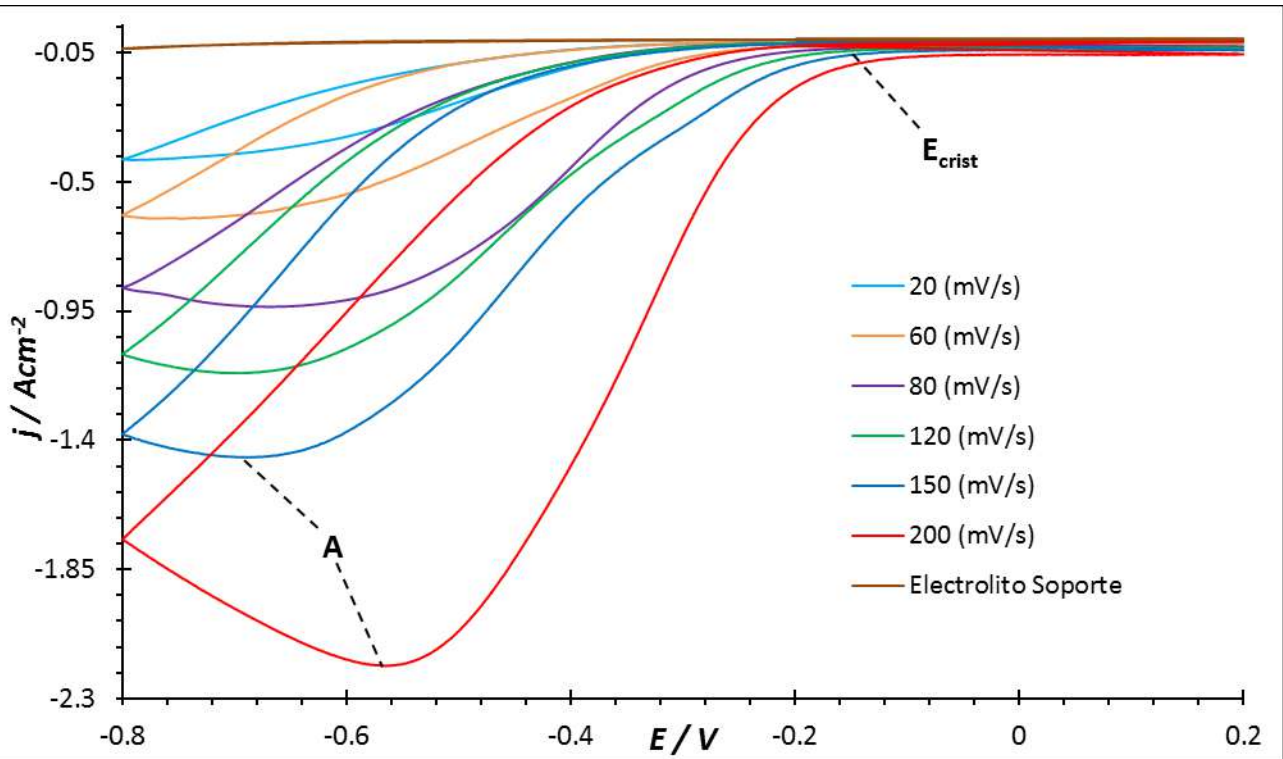
Figura 5.1 Voltamperograma cíclico típico obtenido a partir de los sistemas I y II, utilizando un UME de 10 µm de diámetro, con diferentes velocidades de barrido a 25°C.
