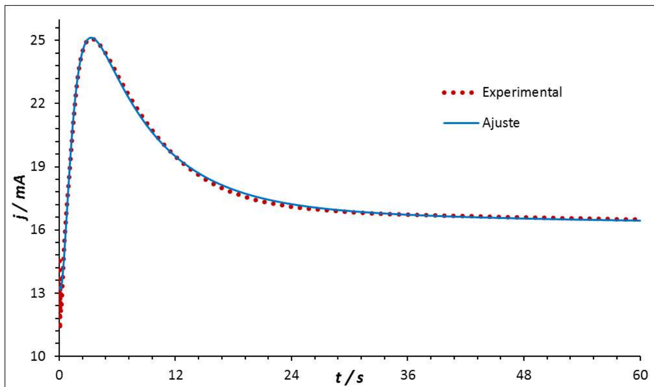
Figura 4.23 Ajuste de un cronoamperograma con potencial de -300 mV mediante el sistema I a 25°C, utilizando el modelo matemático de Palomar-Pardavé et al.
