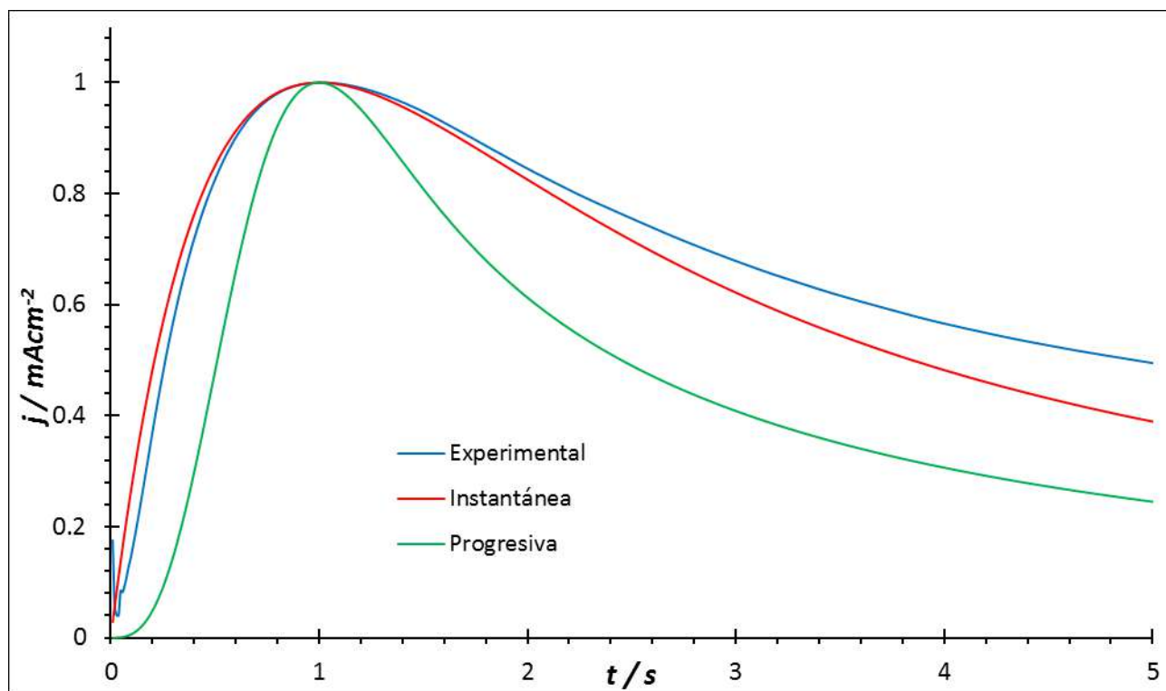
Figura 4.22 Comparación de un transitorio experimental con las curvas teóricas adimensionales.
