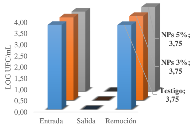
Figura 3. Remoción de Escherichia coli en los pavimentos permeables.
