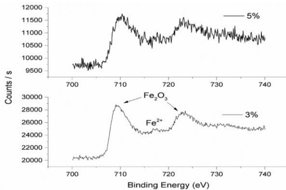
Figura 2. Espectros de XPS de los pavimentos permeables con capa fotocatalítica.
