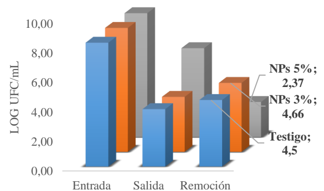
Figura 4. Remoción de Pseudomonas aeruginosa en los pavimentos permeables.
