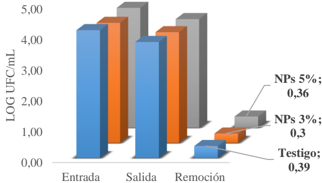
Figura 5. Remoción de Enterococcus faecalis en los pavimentos permeables fotocatalíticos.
