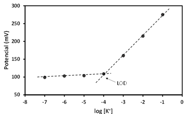
Figura 1. Curva de calibrado potenciométrica, E (vs Ag/AgCl) contra log [K + ]
