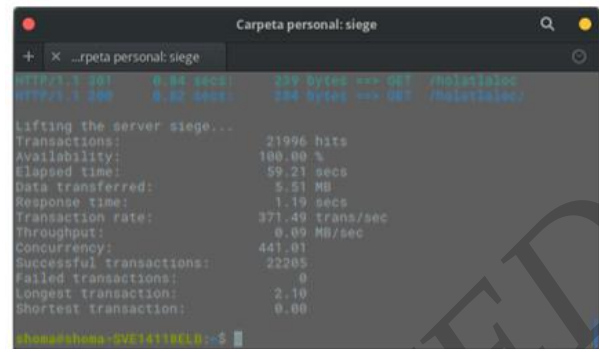
Figura 6. Resultados de la prueba 1.
