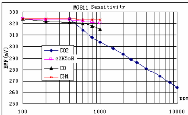
Figura 6.- Gráfica de sensor MG811.
