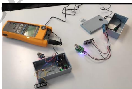
Figura 10.- Armado de cajas de sensores.
