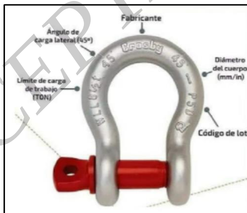
Figura 23. Especificaciones en grilletes
