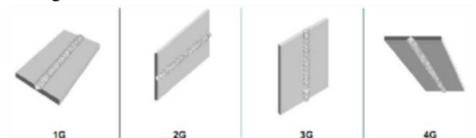
Figura 17. Posiciones de soldadura en ranura (American Welding Society, 2018)
