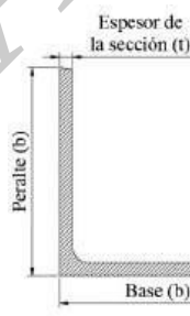
Figura 4. Ángulo de lados iguales (LI)
