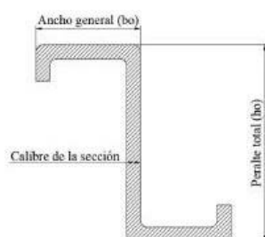
Figura 6. Perfil Z formado en frío (ZF)
