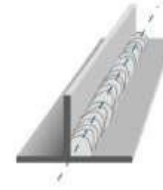
Figura 14. Soldadura en posición 2F (American Welding Society, 2018)
