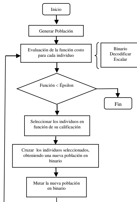
Figura 4: Secuencia de ejecución de un algoritmo genético.
