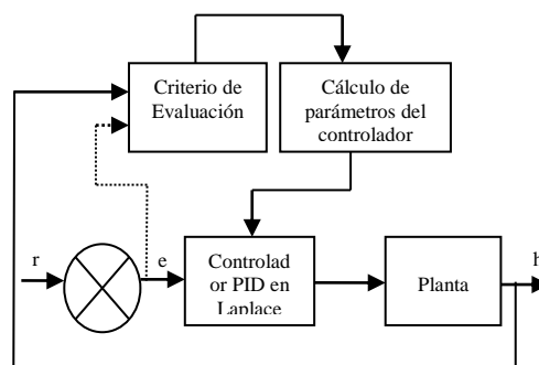
Figura 2: Integración del controlador PID con la planta.
