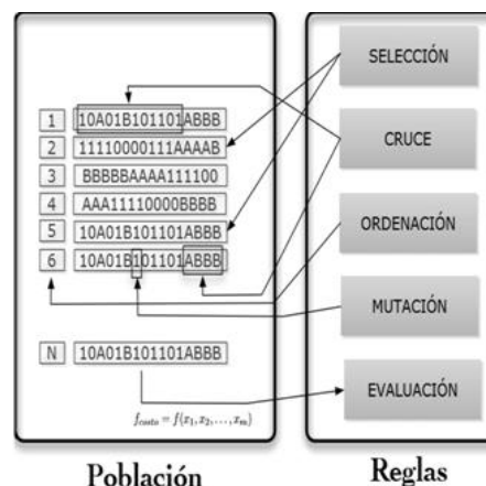
Figura 2: Componentes de un algoritmo genético.
