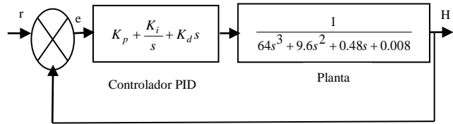
Figura 5: Diagrama de bloques del controlador PID.
